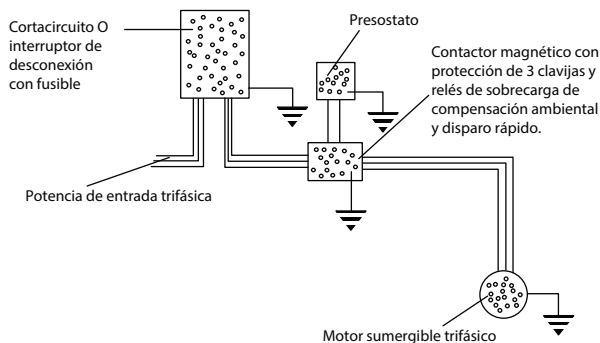
FIGURA 4 - Diagrama de cableado de la bomba de 3 ALAMBRES, trifásica, de 1-1/2 a 10 HP
